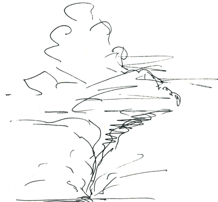
Wirbelsturm
