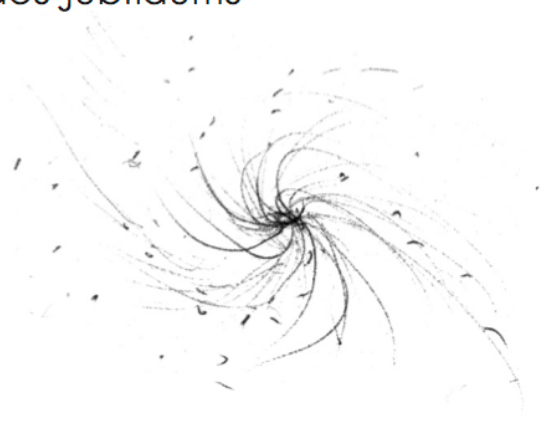
Galaxie
